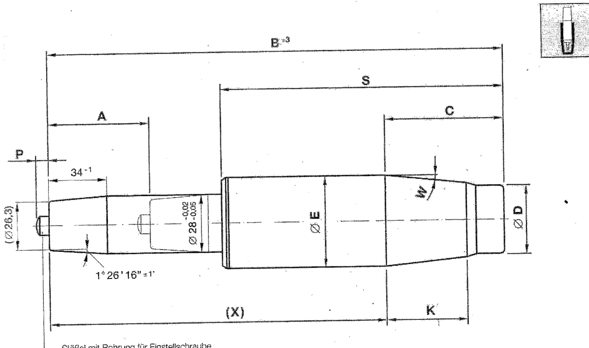
Stößel mit Bohrung für Einstellschraube Release pin suitable for use adjustable screw Bouton de réglage avec perçage pour vis réglage
